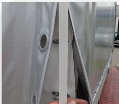
Celní, nedělená plachta z materiálu Mehler, na bocích kapsy proti nadouvání
